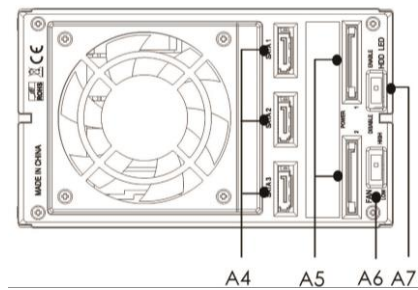
Rückansicht
